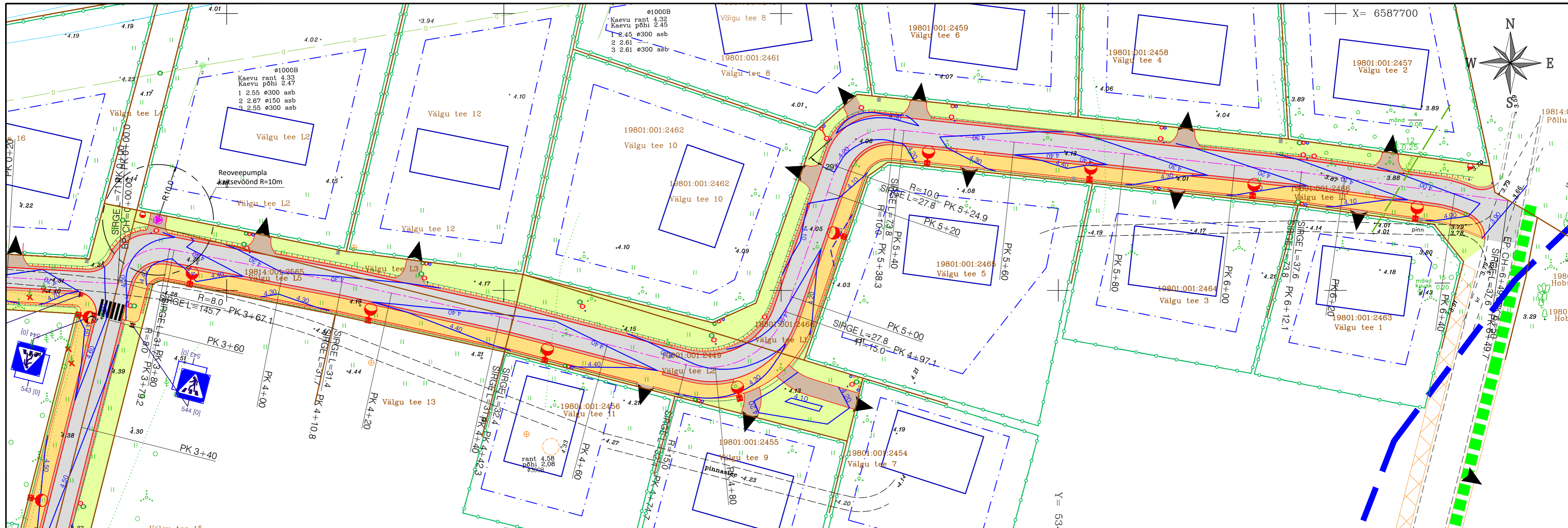
Kiirvool OÜ töö nr. 217/16 tingmärgid: "Ühisveevärgi ja -kanalisatsiooni ehitusprojekt"
